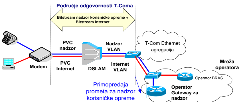
Slika 29. Veleprodajni širokopojsni pristup za pružanje usluge nadzora korisničke opreme preko ADSL/VDSL pristupa na DSLAM razini
