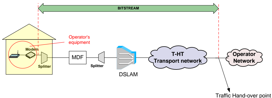
Slika 31. Koncept posebnog virtualnog kanala za Podatkovnu uslugu
