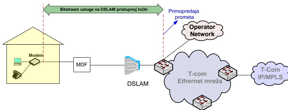
Slika 7. Veleprodajni širokopojasni pristup za pružanje Internet usluge na DSLAM razini u slučaju kada krajnji korisnik ostvaruje Osnovni pristup mreži putem usluge HT-a
