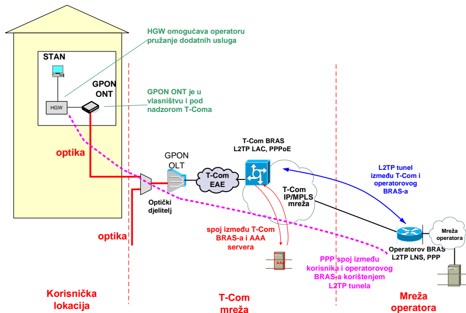
Slika 2. Način realizacije usluge veleprodajnog širokopolasnog pristupa za Internet uslugu na temelju FTTH rješenja na IP razini
